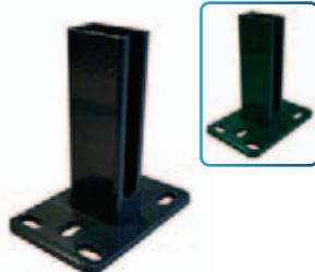
Montagefüße für Pfosten 60 x 40 mm zum Aufschrauben auf festem und ebenen Untergrund. 150 x 100 x 8 mm
