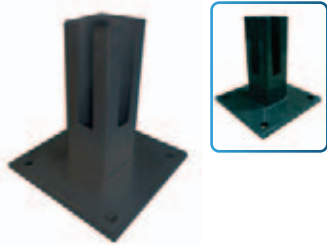
Montagefüße für Eck-Pfosten 60 x 60 mm zum Aufschrauben auf festem und ebenen Untergrund. 150x150x8 mm
