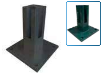
Montagefüße für Eck-Pfosten 60 x 60 mm zum Aufschrauben auf festem und ebenen Untergrund. 150 x 150 x 8 mm
